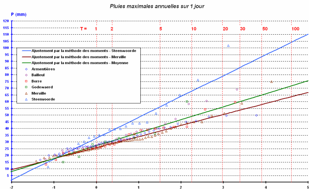
Figure 13 : Ajustement de Gumbel des différents postes pluviométriques.
