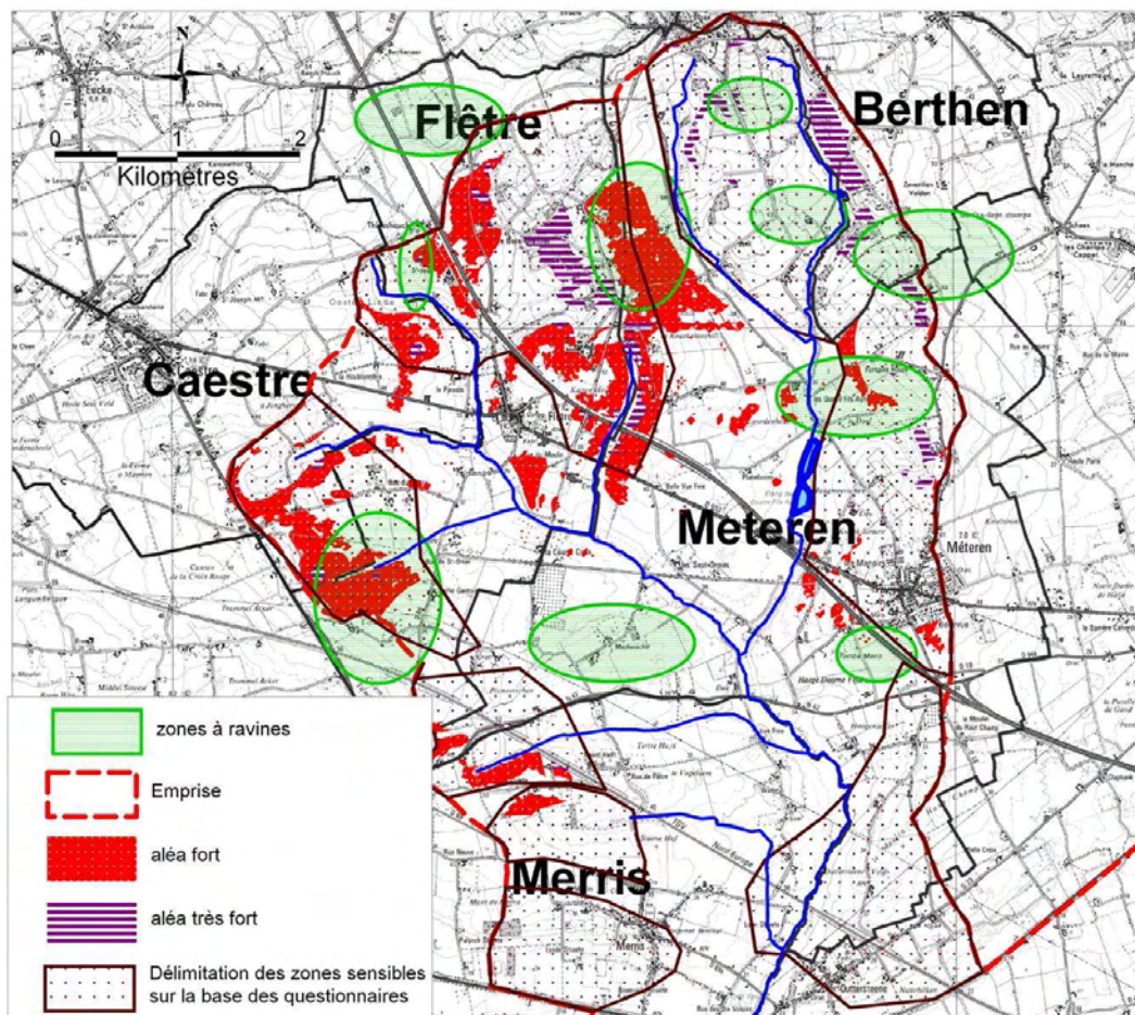
Figure 37 : Comparaison entre la cartographie des secteurs sensibles à l'érosion et les secteurs recensés lors de l'enquête de phase 1.
