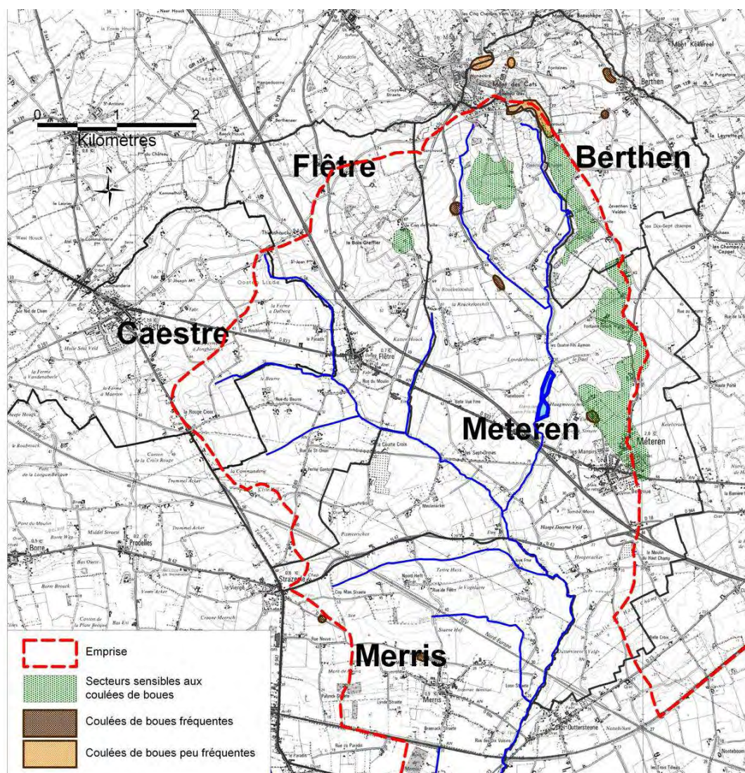
Figure 38 : Comparaison entre la cartographie de la sensibilité aux coulées de boues et les coulées de boues observées.
