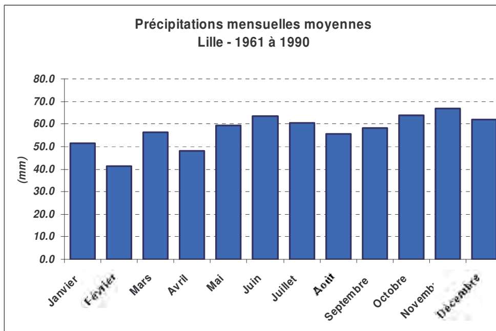
Figure 11 : Précipitations mensuelles moyennes à Lille.
