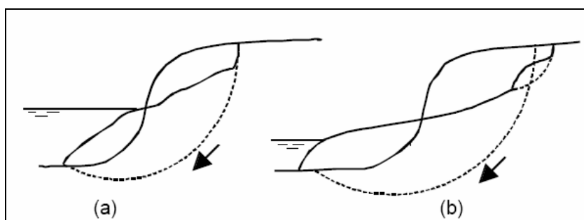
(a : rupture circulaire d'un talus instable ; b : rupture circulaire du même talus après une décrue plus forte, et ruptures secondaires)
